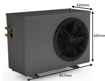
Unité extérieur
